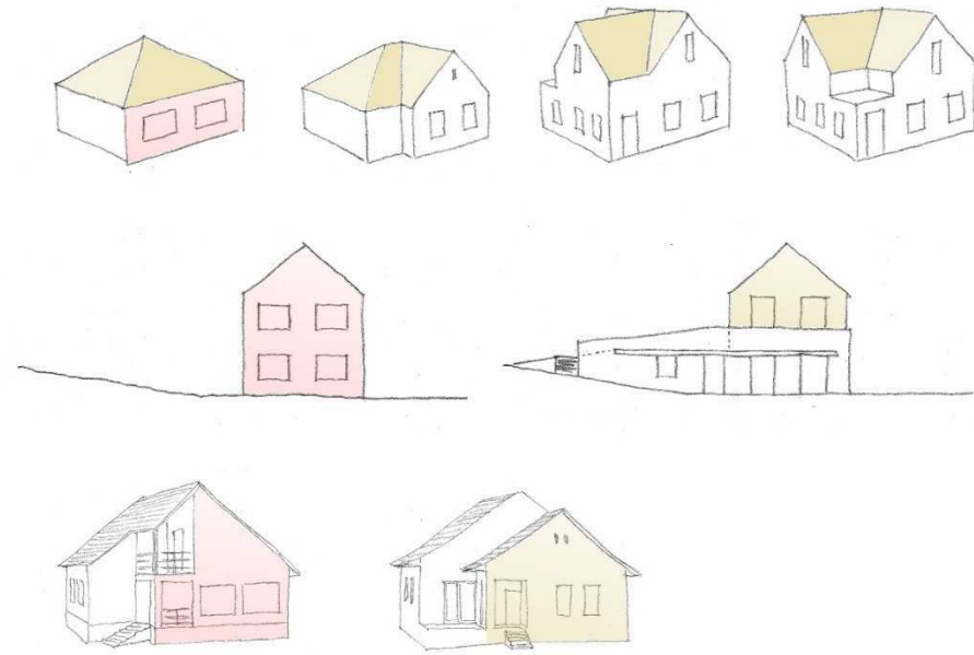
Néhány példa meglévő épületek átalakítására a tömegek, tetőidomok tagolásával. Érdemes a hagyományos házforma megidézésére, és emellett a hagyományos - max. 7,50 m épületszélességre törekedni az utcai homlokzatnál
